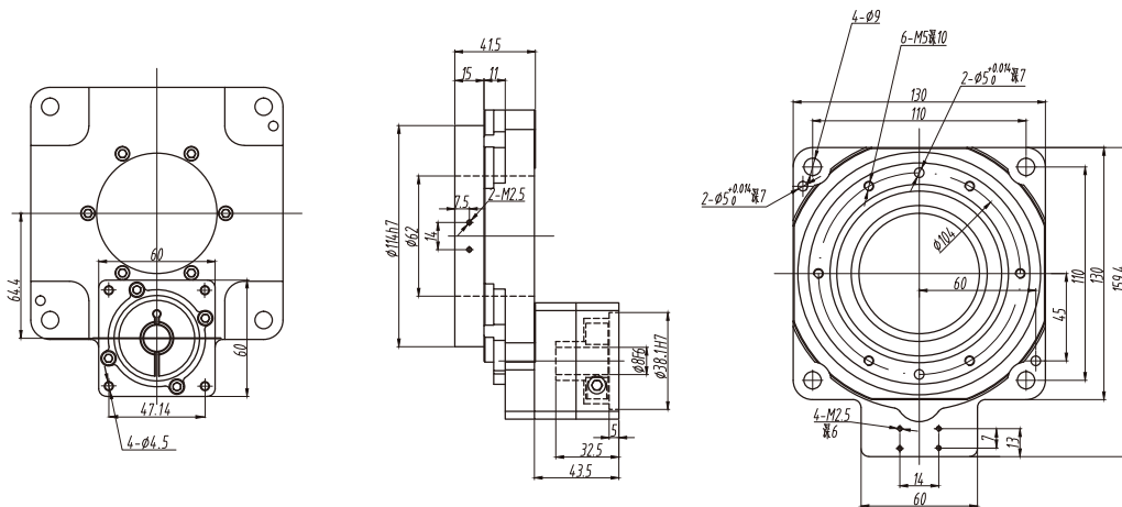
SH130-10-S(尺寸圖)
